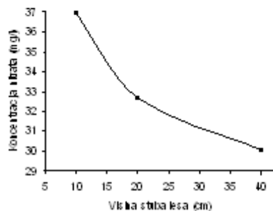
Slika 1. Konzentracije nitrata u odnosu na vreme potrebno da rastvor istekne pri kontinualnom protoku i u odnosu na visinu stuba peska i lesa
