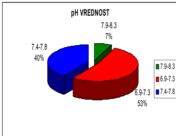
Slika 2. Ciklogrami hemijskog sastava podzemnih voda
